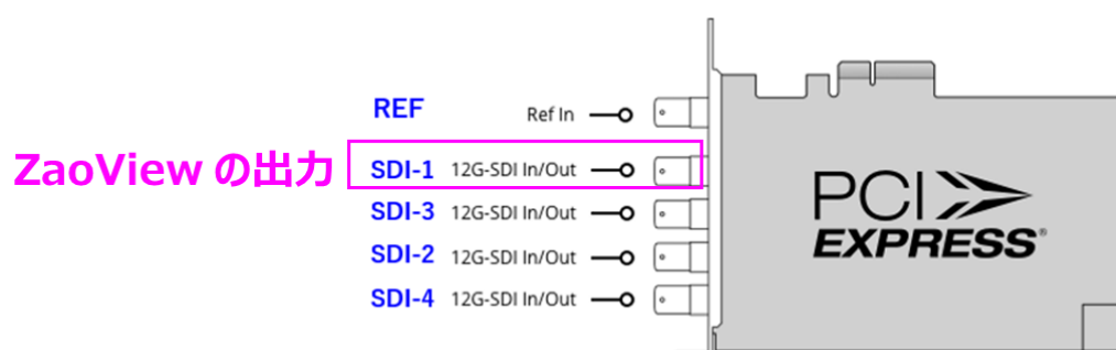
図 3-48 DeckLink 8K Pro の SDI 外部モニタとの接続ポート
