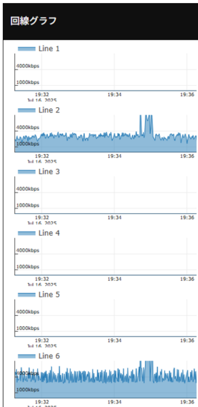
図 113 マルチリンク対応送信機の回線ビットレートグラフ
